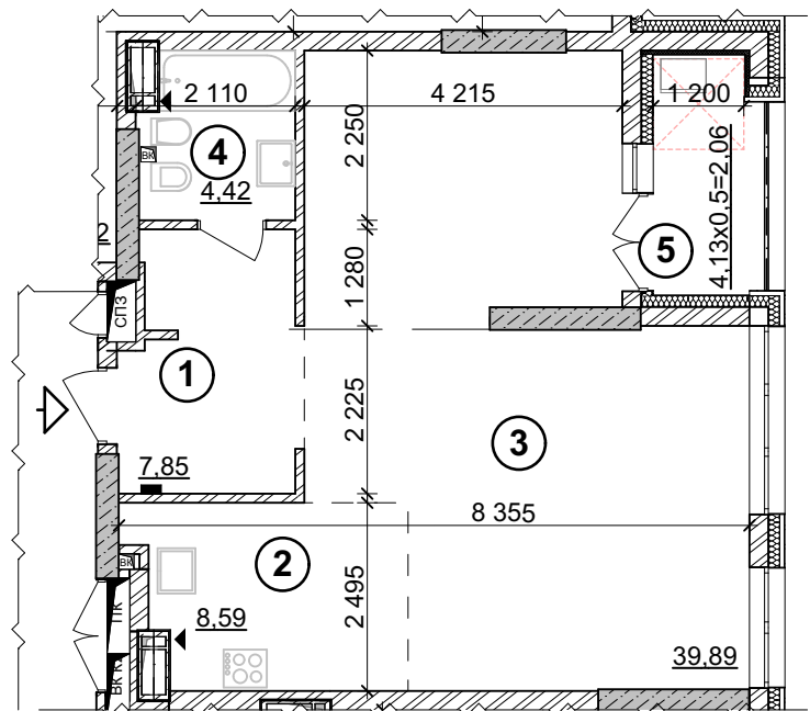
План 7-го поверху
